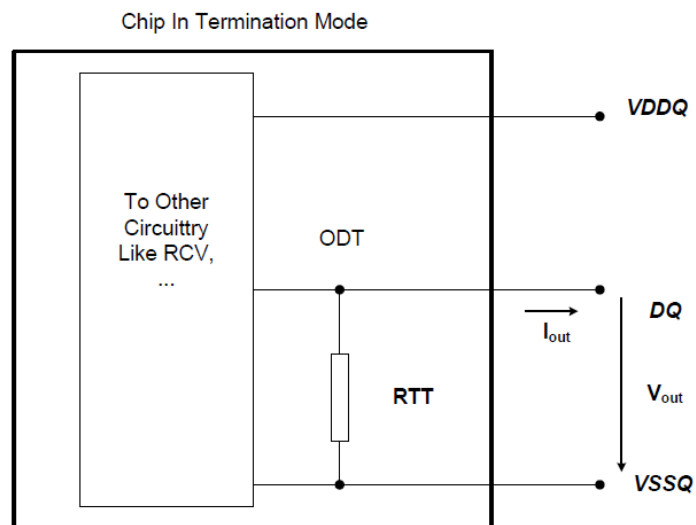
Figure 143 - DQ On Die Termination
