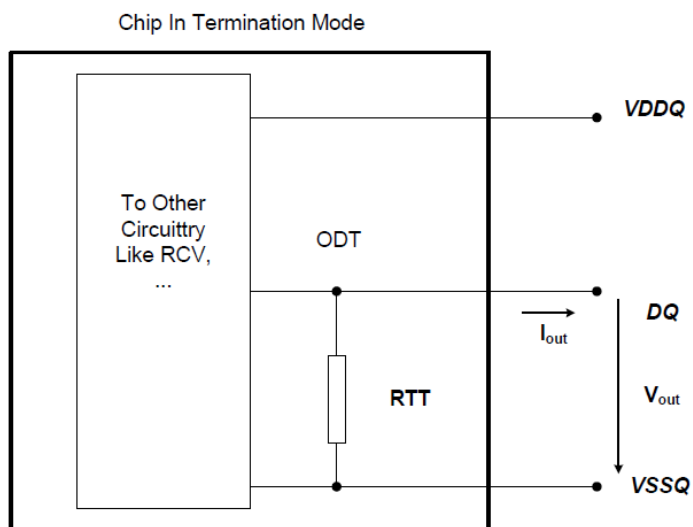
Figure 144 - DQ On Die Termination
