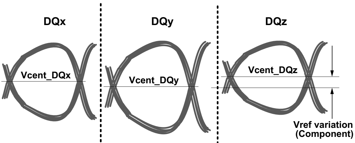
Figure 187 - Across pin Vref DQ voltage variation
